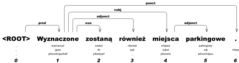
Figure 7: Dependency tree of Wyznaczone zostaną również miejsca parkingowe . (Eng. ‘Parking spaces will also be designated.’)
