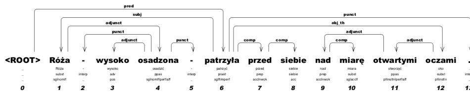
Figure 4: Dependency tree of Róża – wysoko osadzona – patrzyła przed siebie nad miarę otwartymi oczami . (Eng. ‘Rose – placed highly – was looking straight ahead with her eyes open too widely.’)
