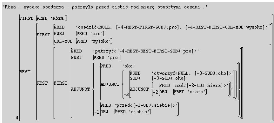
Figure 2: The FRAGMENT parse of Róża – wysoko osadzona – patrzyła przed siebie nad miarę otwartymi oczami. (Eng. ‘Rose – placed highly – was looking straight ahead with her eyes open too widely.’)
