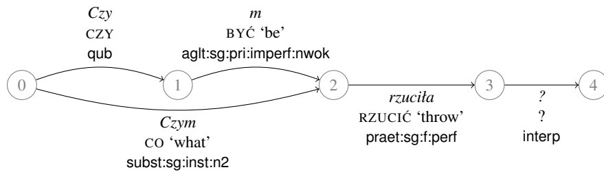
Figure 1: Morfeusz analysis of Czym rzuciła?
