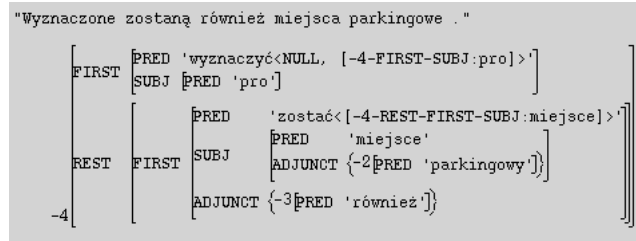
Figure 6: The FRAGMENT parse of Wyznaczone zostaną również miejsca parkingowe . (Eng. ‘Parking spaces will also be designated.’)
