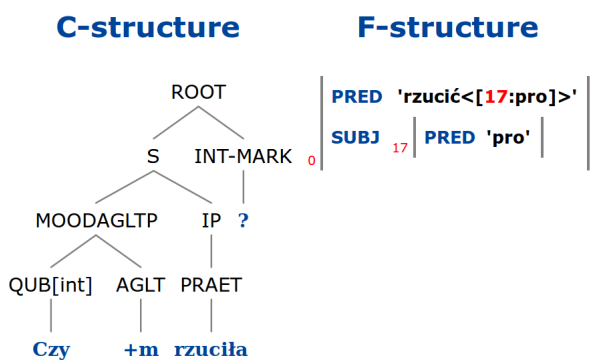
Figure 3: Czym rzuciła? – structures for interpretation (2), Morfeusz-based tokeniser.
