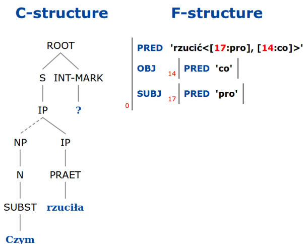
Figure 4: Czym rzuciła? – structures for interpretation (1).
